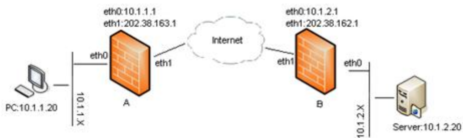
图 56-1 案例组网图
