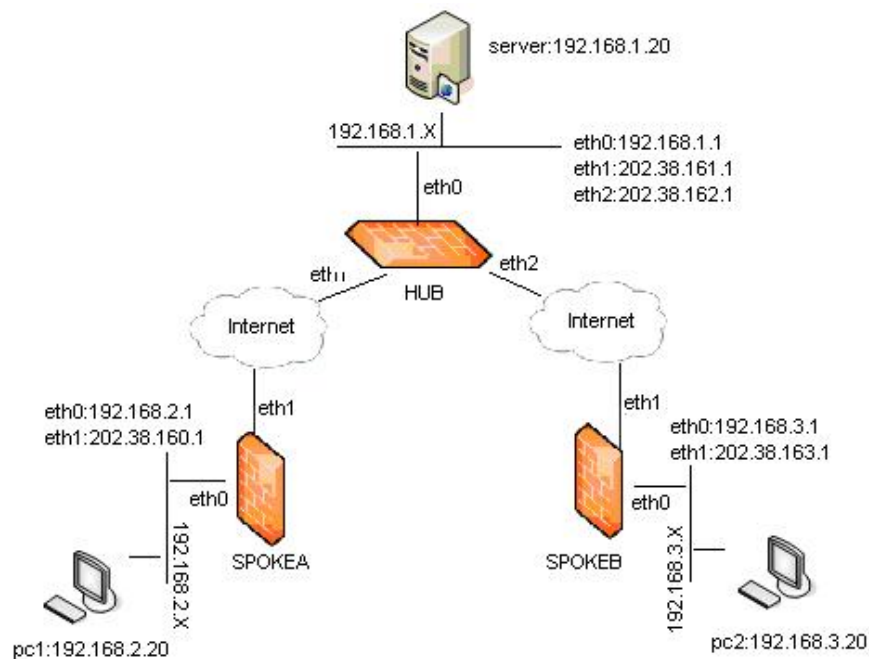
图 56-2 案例组网图
